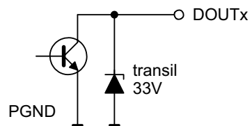
Obr. 1. Zjednodušené schéma vnitřních obvodů digitálních výstupů.
