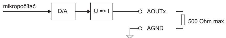
Obr. 1. Zjednodušené schéma vnitřních obvodů analogových výstupů. (výstupní proud 0~20 mA; maximální napětí 10 V)
