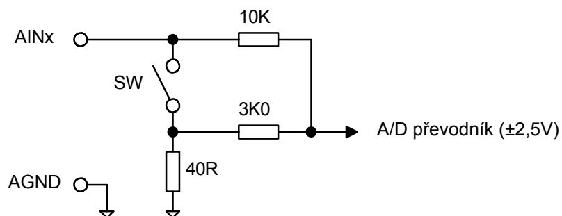
Obr.2. Schéma připojení napěťových signálů (spínač rozepnutý) a proudových signálů (spínač sepnutý).
