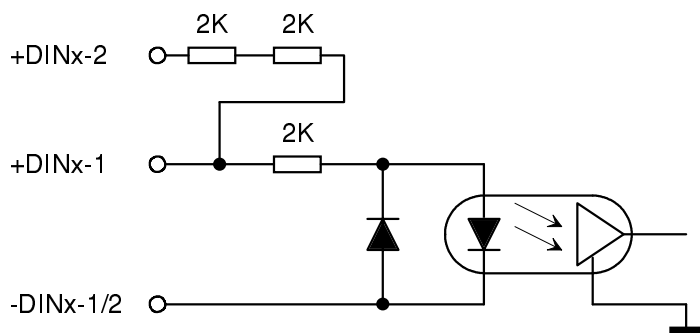
Obr.2A. Zjednodušené schema obvodů digitálních vstupů modulu MU-631.
