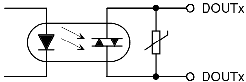
Obr.3B. Zjednodušené schema obvodů digitálních výstupů modulu MU-632.
