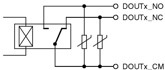
Obr.3A. Zjednodušené schema obvodů digitálních výstupů modulu MU-631.
