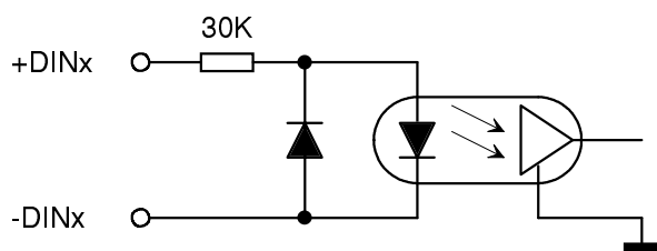
Obr.2B. Zjednodušené schema obvodů digitálních vstupů modulu MU-632.
