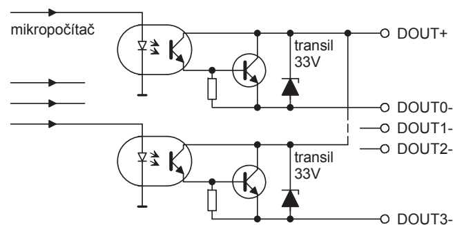
Obr. 3. Zjednodušené schéma vnitřních obvodů digitálních výstupů.
